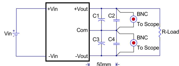
EC2SAW8 Single Output Module
