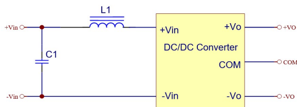
EC2SAW8 Dual Output Module
