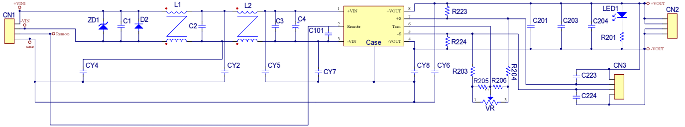
Figure1 Schemati
